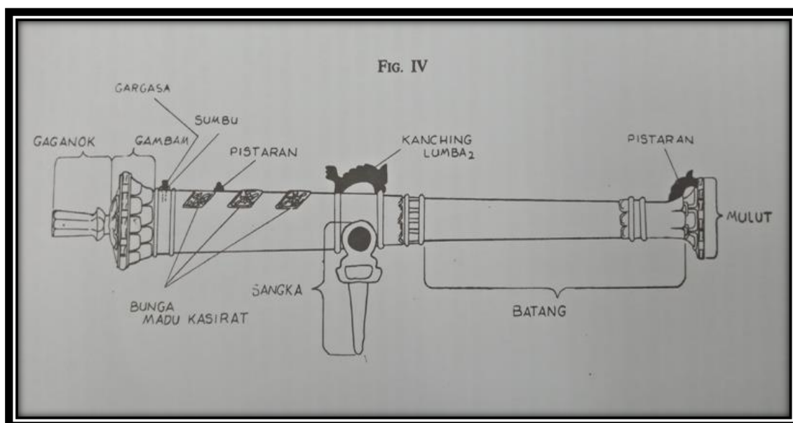
Rajah 1. Nama-nama pada bahagian meriam Melayu iaitu lela dan rentaka Sumber: P. M. Sharifuddin 2012
