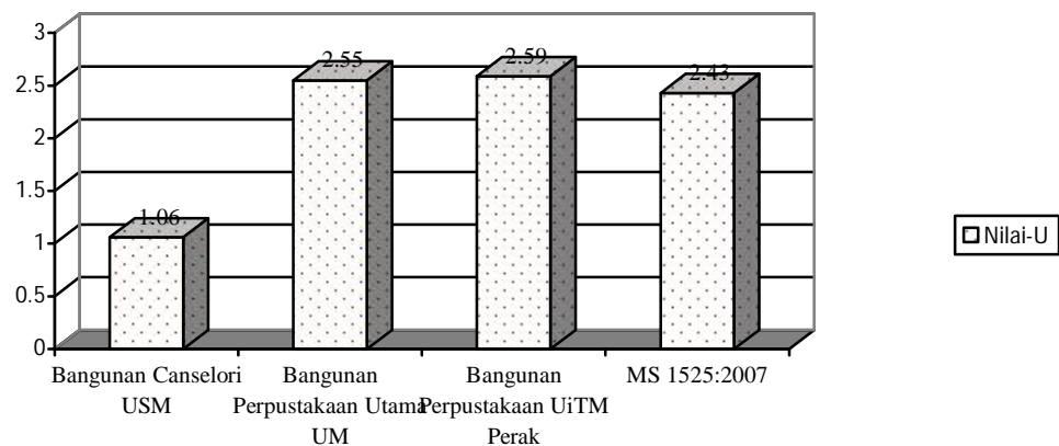
Carta 2: Perbezaan Antara Nilai-Nilai U-Value
