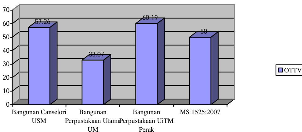
Carta 1: Perbezaan Antara Bangunan Canselori Universiti Sains Malaysia dengan Garis Panduan MS 1525:2007
